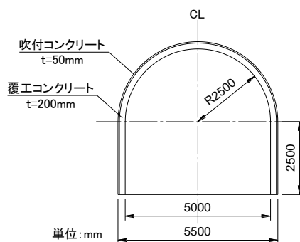
図 1 対象とする坑道（主要坑道の例）
